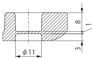
取付穴断面図
