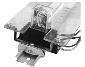
[リレー 取付例]
