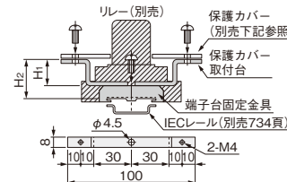
[取付方法]
