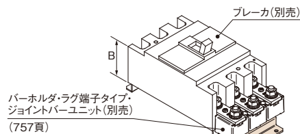
〔BP34-LT□25D取付例〕
