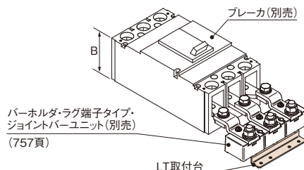
〔BP34-LT□40(W)D取付例〕
